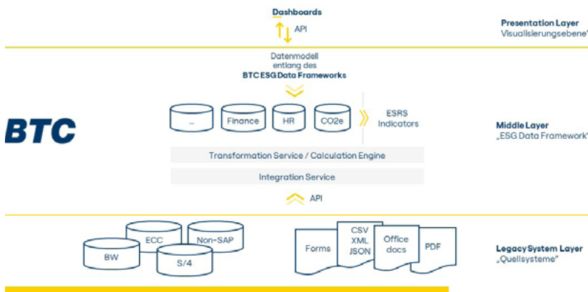
Abb. 2: Aufbau des BTC Data Hubs inkl. ESG Data Framework
